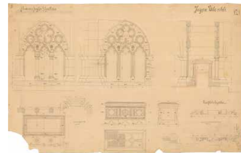
III. Béla tervezett, de meg nem valósult altemplomi síremlékének terve, Wagner Ferenc, 1887 (Kiscell É)
